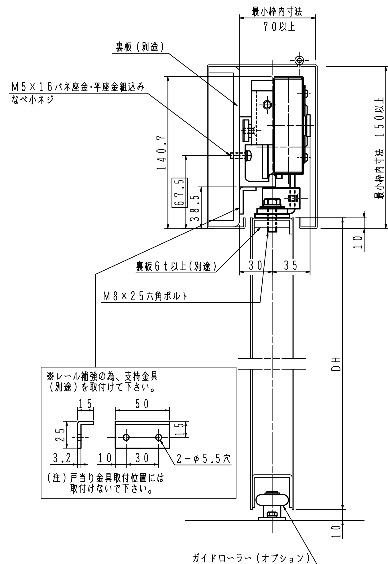
左側面図
