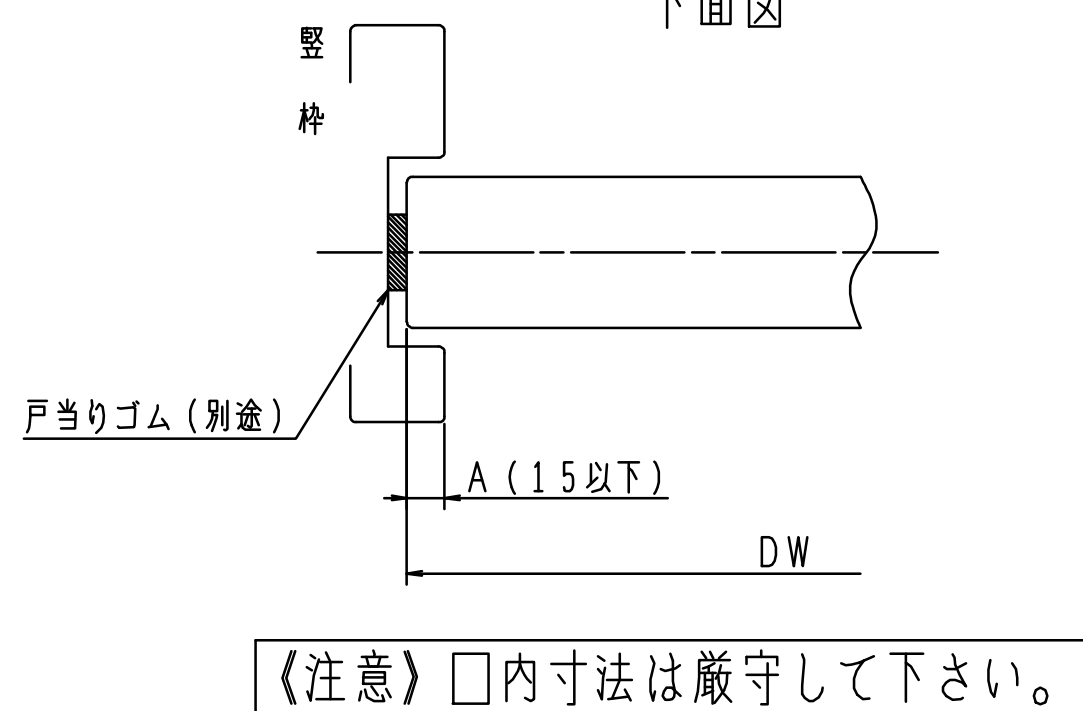
下面図
