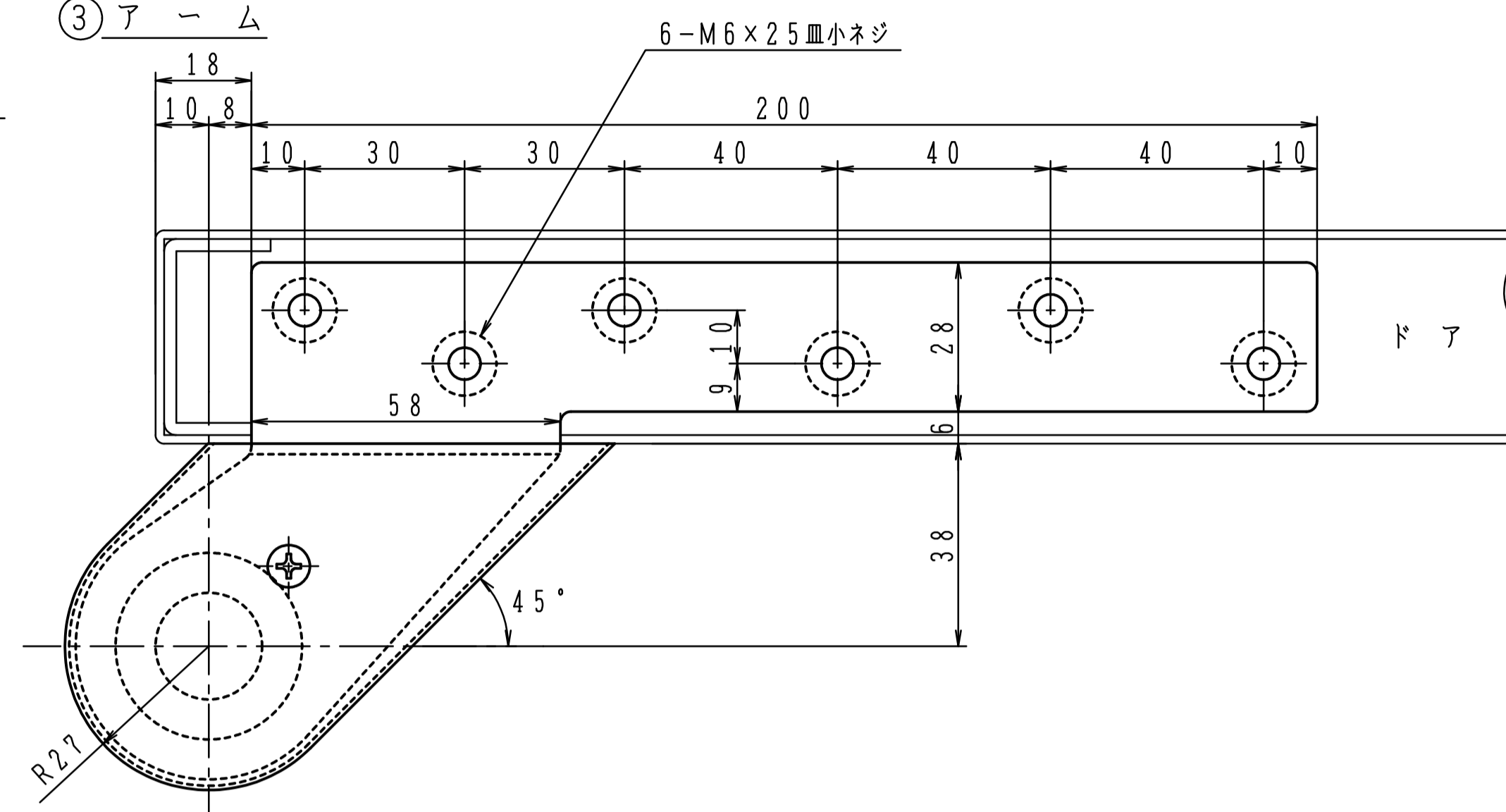
③ アーム
