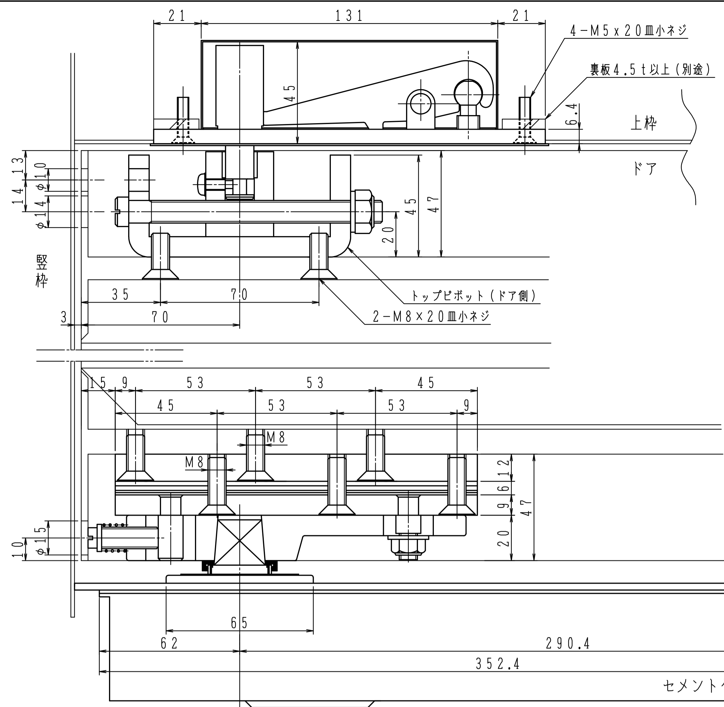
トップピボット (上枠側)
