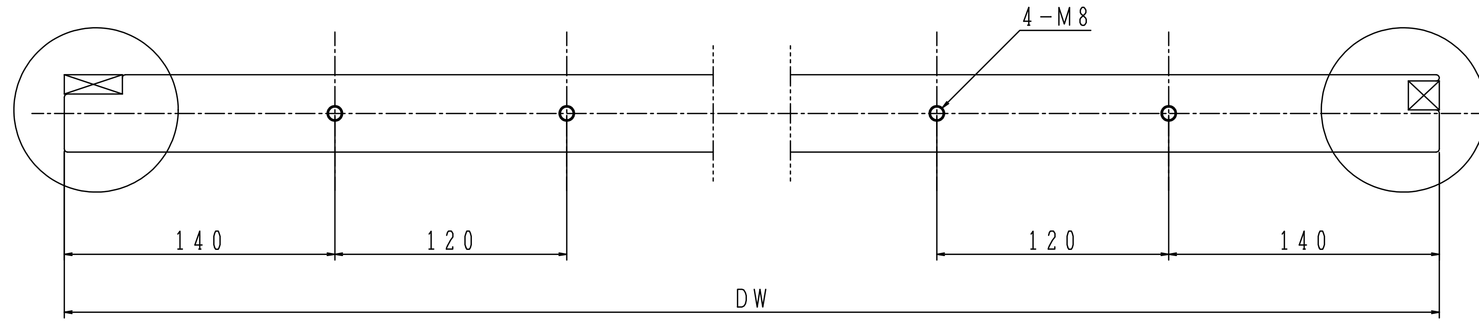
扉上面図
