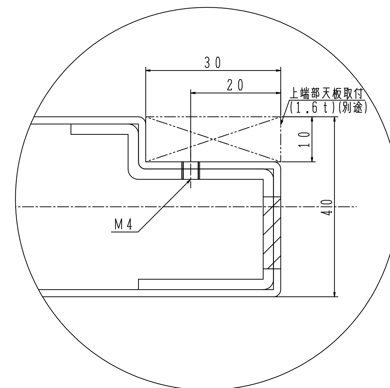
戸尻側断面図
