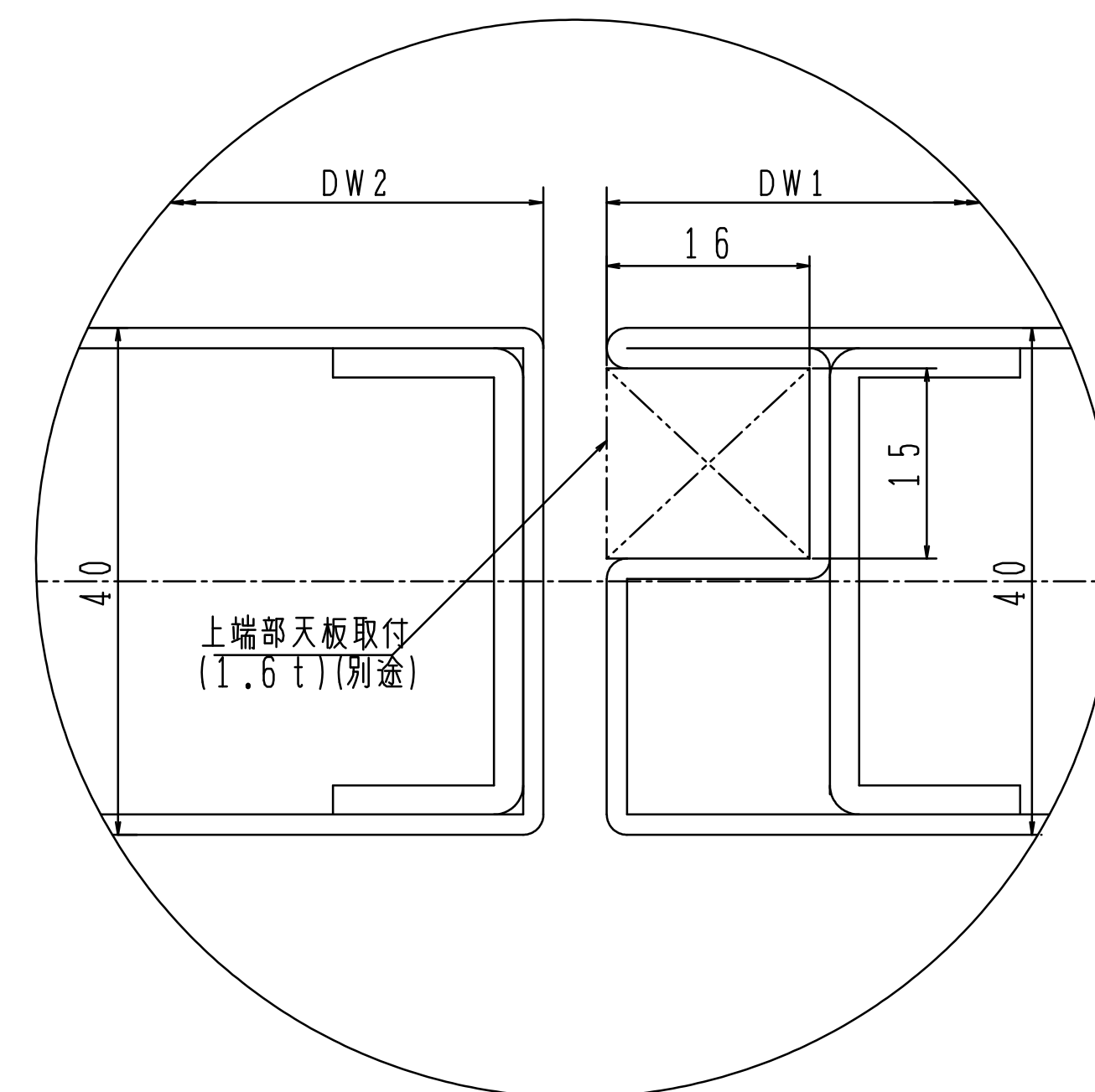
召合せ部断面図
