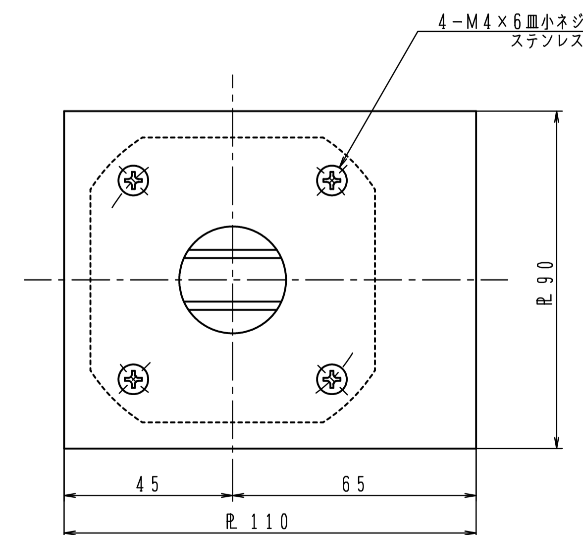
④ 床面軸座
