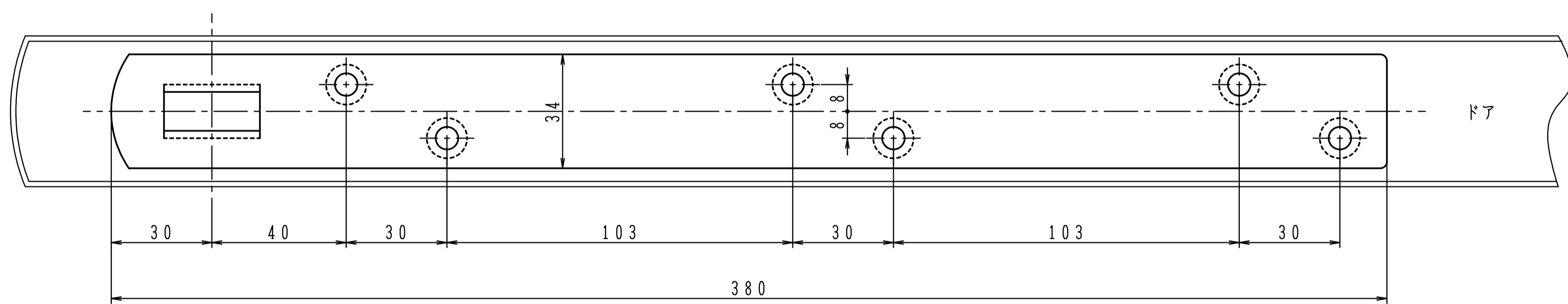
③ アーム
