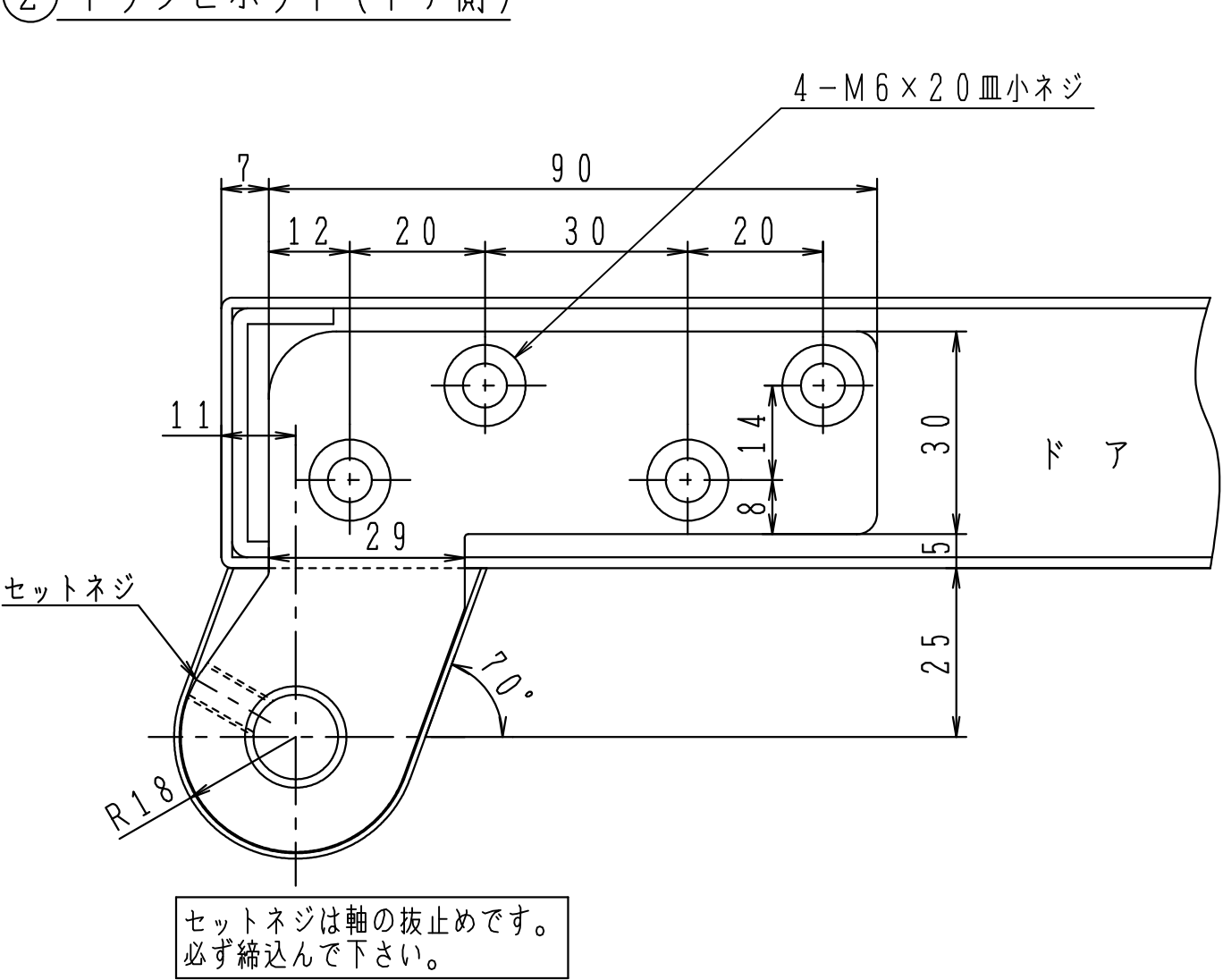
② トップピボット（ドア側）
