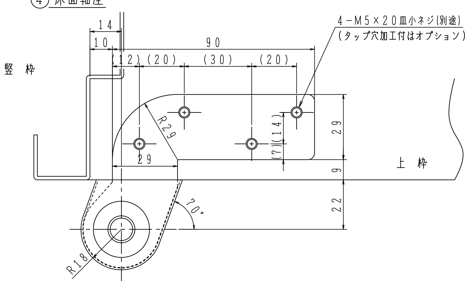
④ 床面軸座
