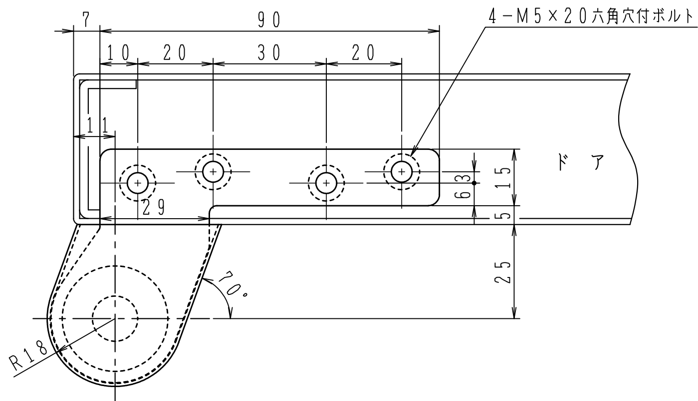
③ アーム
